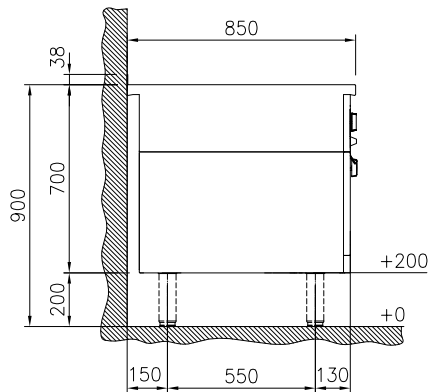
Zij aanzicht
